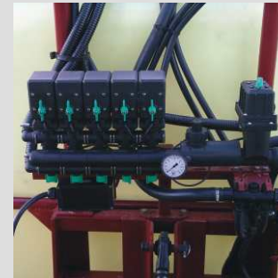
Distribuidor eléctrico HARDI con regulación volumétrica.
